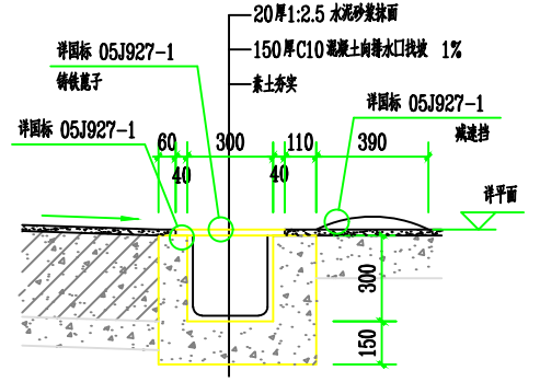
300截水边沟
