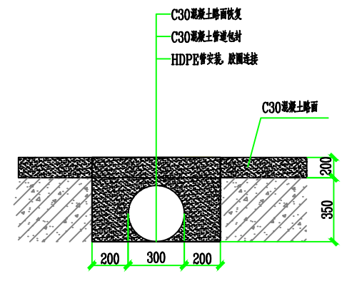
HDPE管截面图
