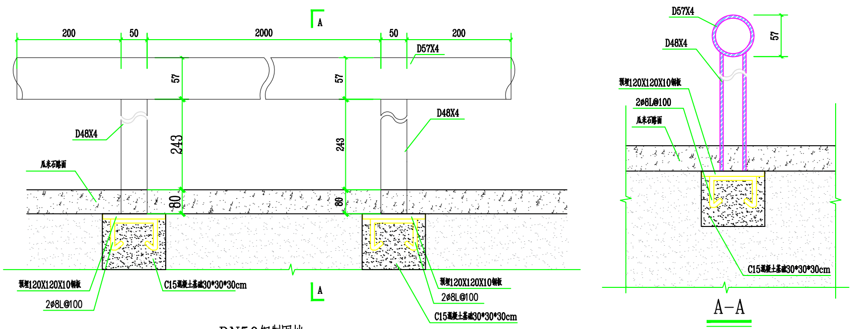
DN50钢制围挡
